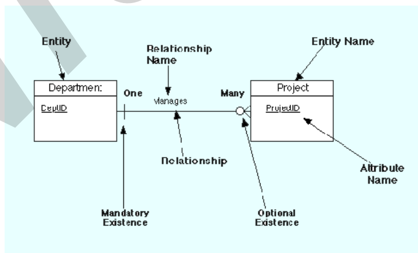
Figure 2.1 ER Notation
